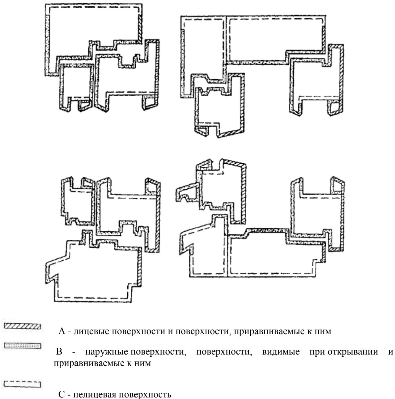
Рисунок 8 - Примеры определения видов поверхностей деталей
