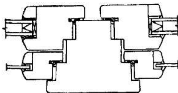
Рисунок 3 - Примеры конструктивных решений импостных и безимпостных притворов оконных блоков спаренной конструкции (вариант распашного открывания)
