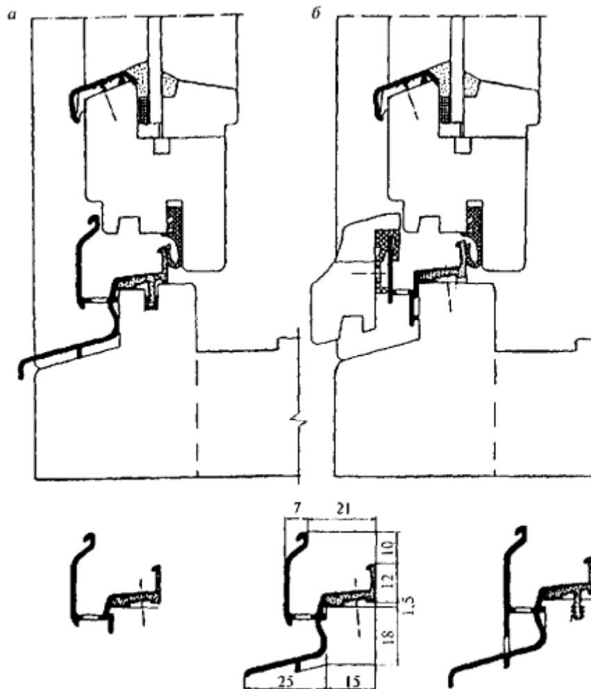
Рисунок 12 - Примеры конструкций дождезащитных профилей:
