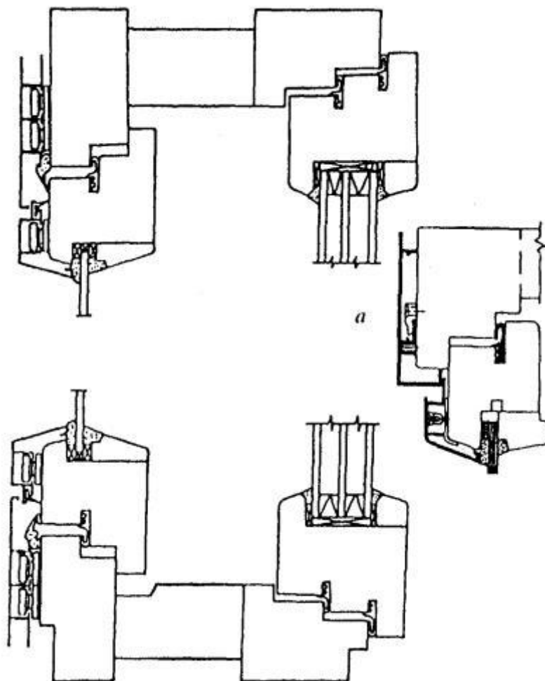
a - вариант конструкции облицовки
