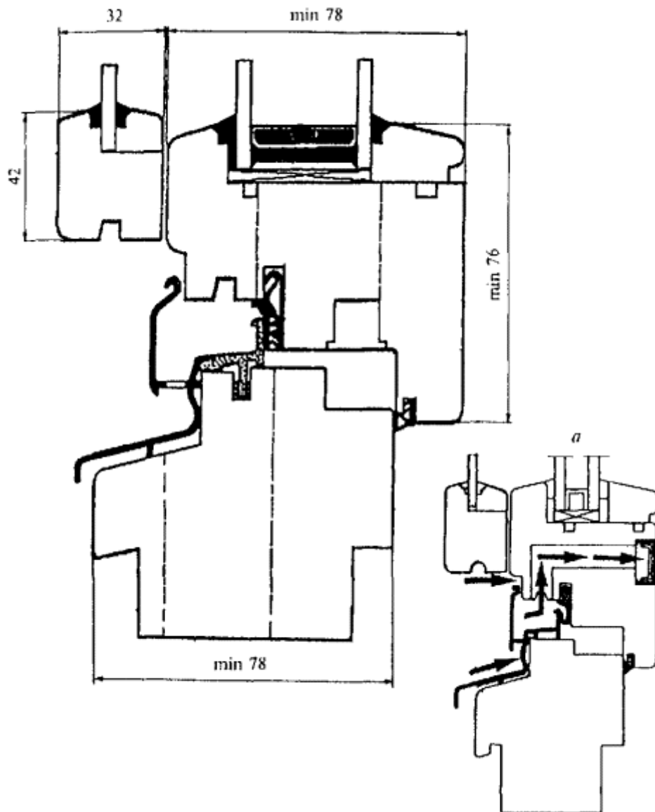
a - вариант установки климатического клапана
